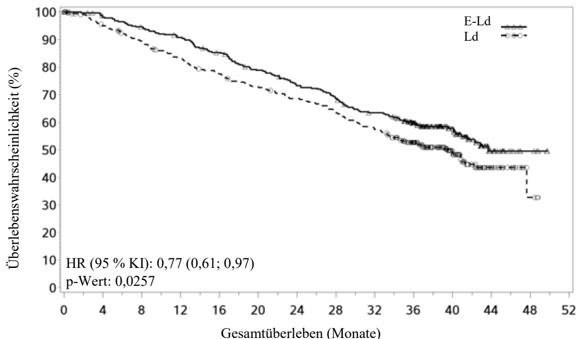
Abbildung 2: CA204004 Gesamtüberleben
