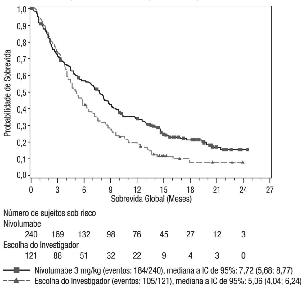
Figura 17: Curvas de Kaplan-Meier de SG (CA209-141)
