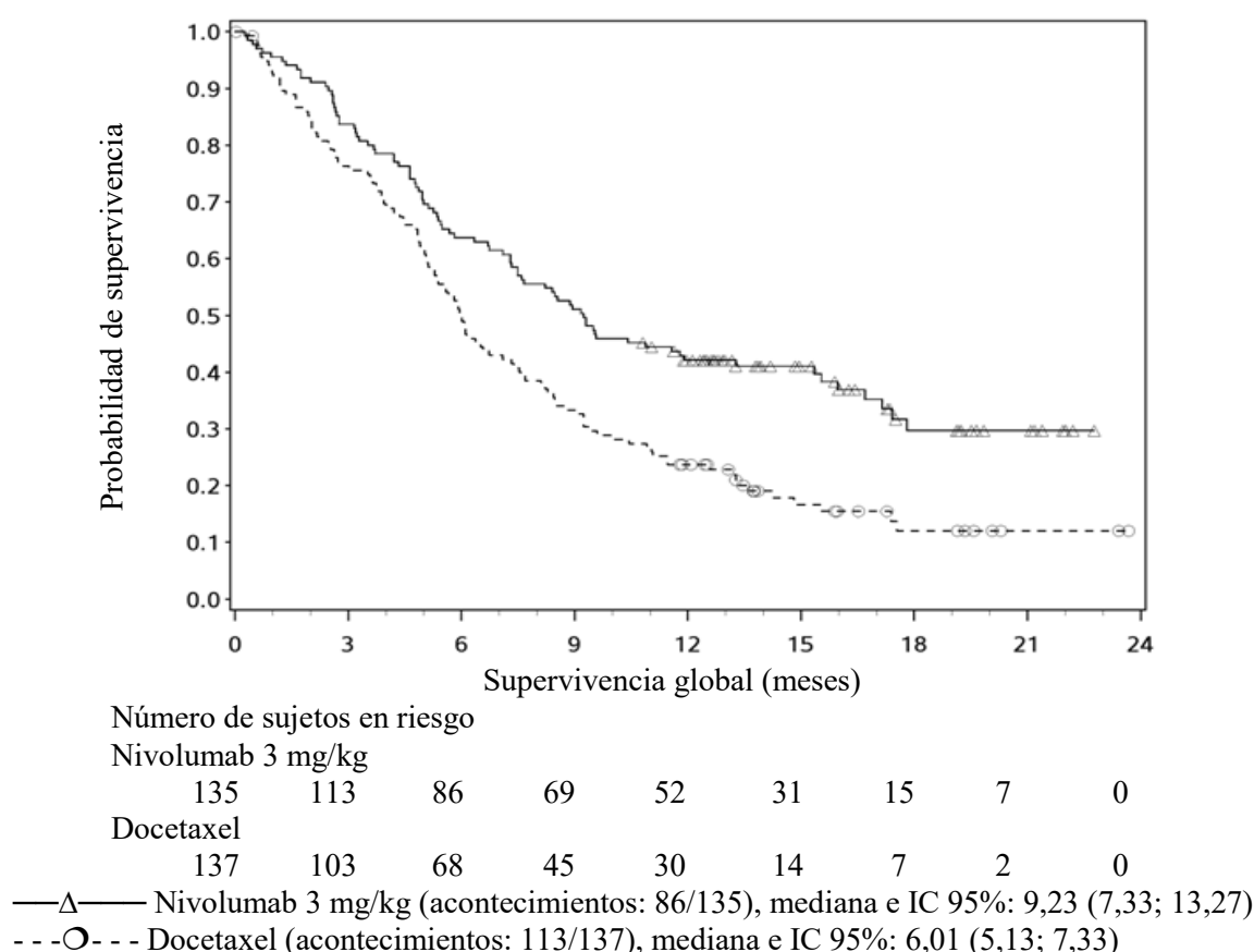
Figura 9: Curvas de Kaplan-Meier de SG (CA209017)
