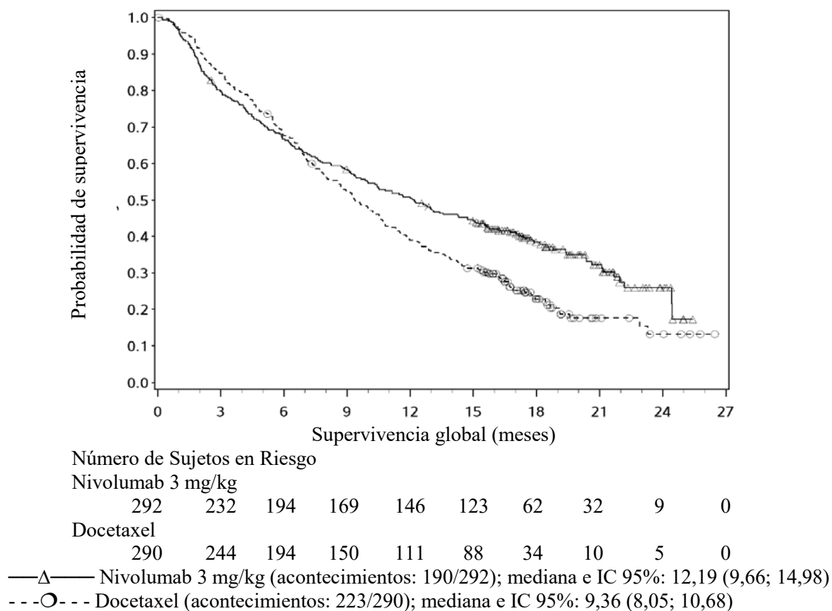
Figura 10: Curvas de Kaplan-Meier de SG (CA209057)
