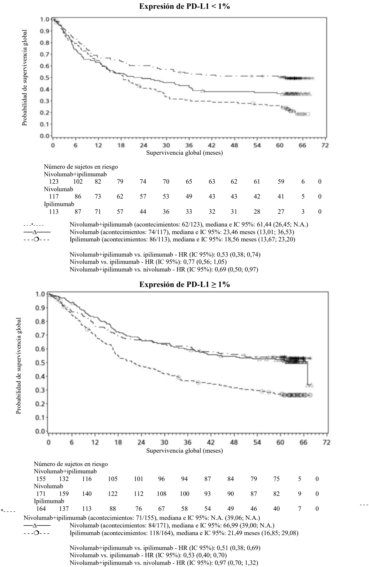
Figura 7: Supervivencia global según la expresión de PD-L1: cut off del 1% (CA209067) - Seguimiento mínimo de 60 meses
