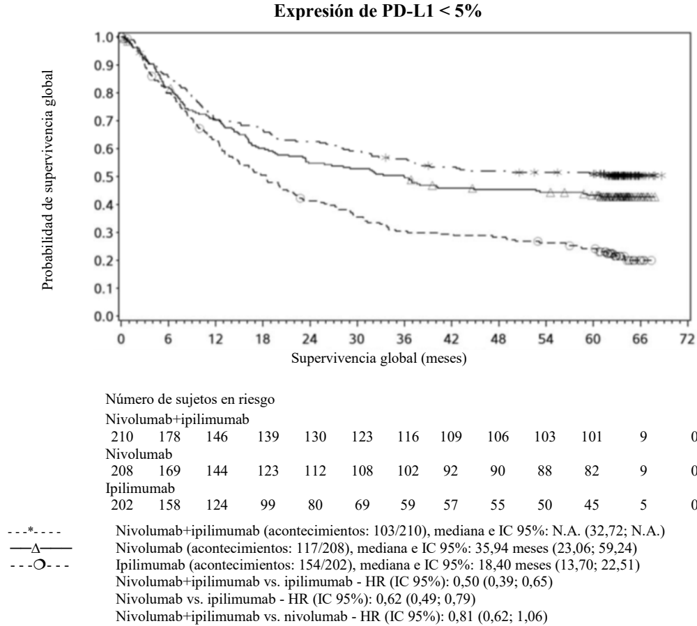
Figure 6: Supervivencia global según la expresión de PD-L1: cut off del 5% (CA209067) - Seguimiento mínimo de 60 meses
