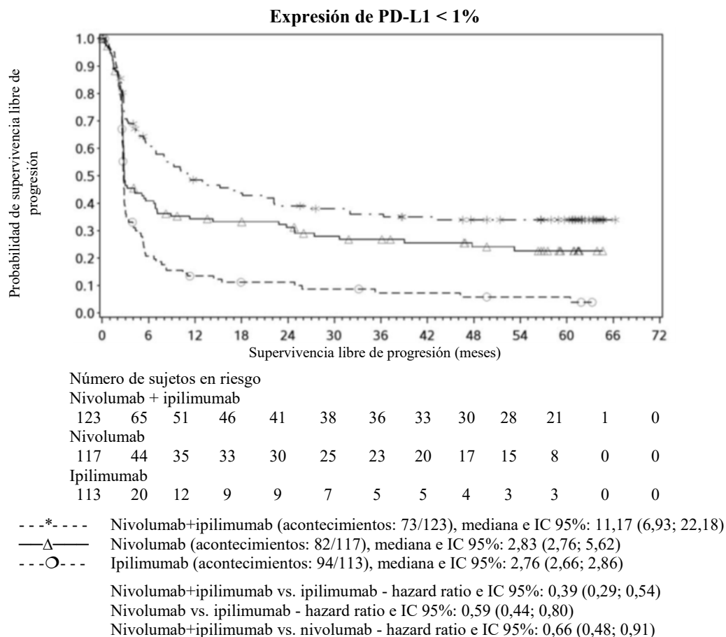
Figura 4: Supervivencia libre de progresión según la expresión de PD-L1: cut off del 1% (CA209067)
