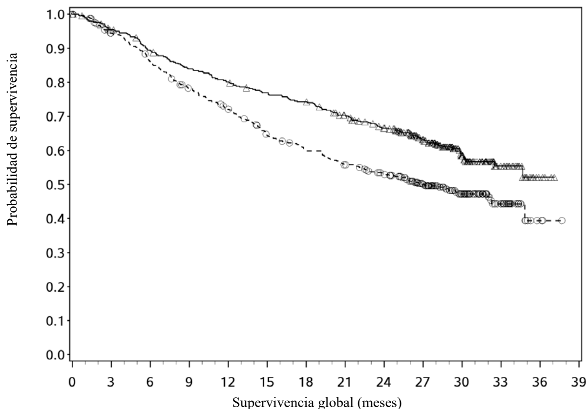
Figura 12: Curvas de Kaplan-Meier para SG en pacientes de riesgo intermedio/alto (CA209214)
