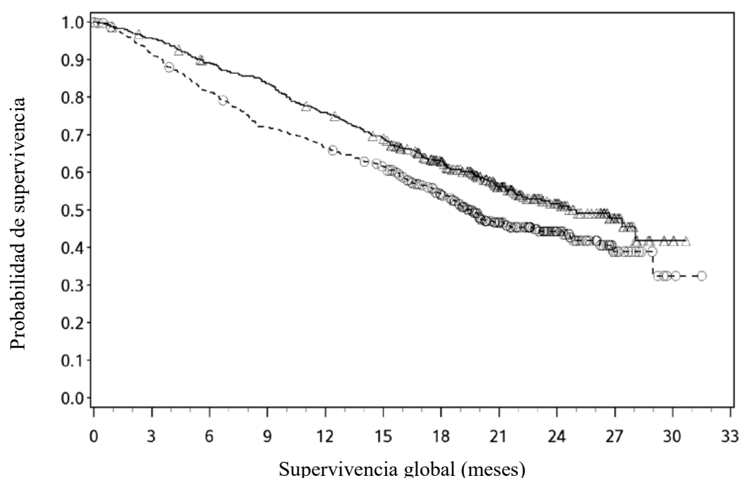
Figura 11: Curvas de Kaplan-Meier de SG (CA209025)
