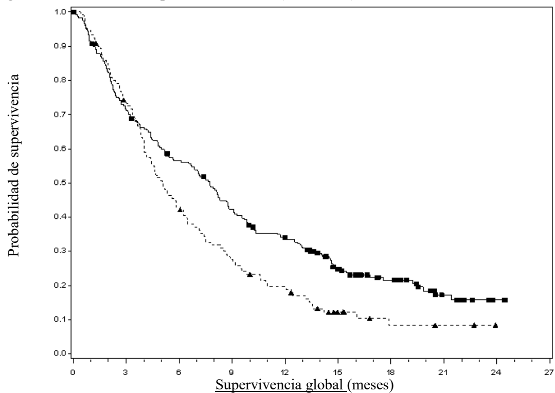
Figura 13: Curvas de Kaplan-Meier de SG (CA209141)
